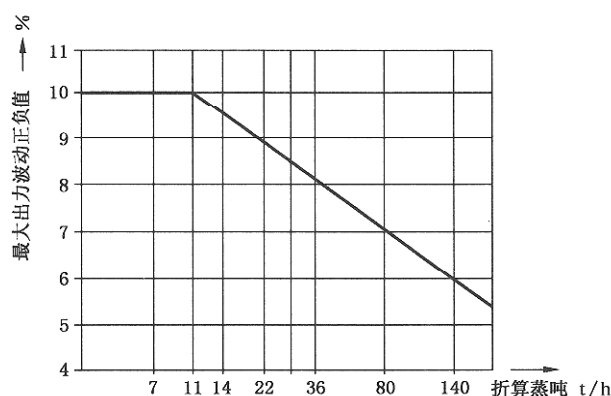
图 1 最大允许的出力波动值
